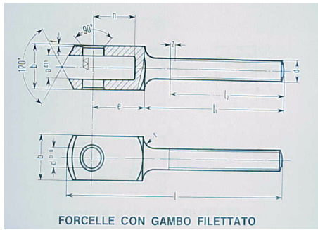
FORCELLE CON GAMBO FILETTATO
