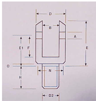
Forcelle FE quote sottoindicate mat. 9SmPb23 R> 50Kg./mm
