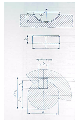
Linguetta a Disco UNI 6606- DIN 6888 toll.h9
