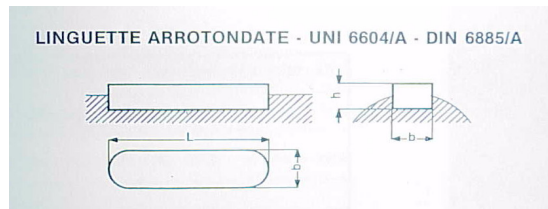
Linguetta tipo A(arrotondate) NON UNIFICATE
